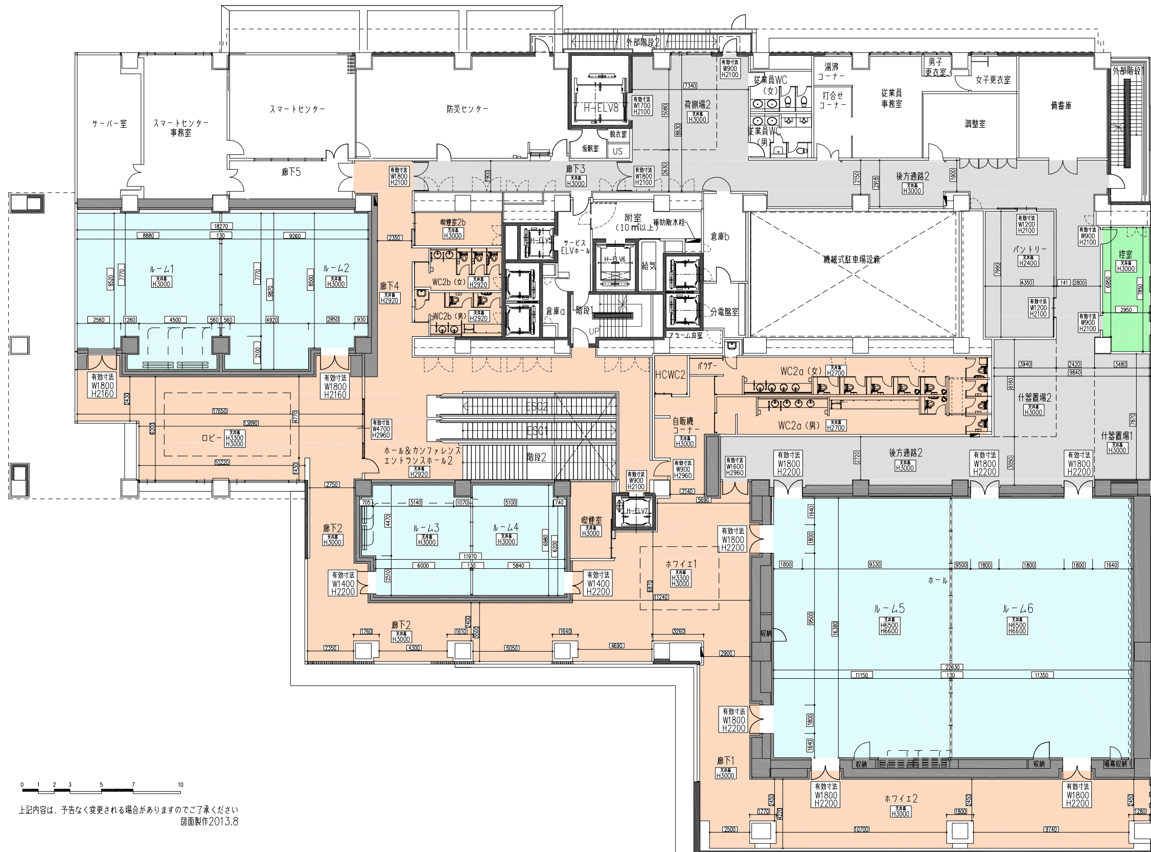
2階平面図
